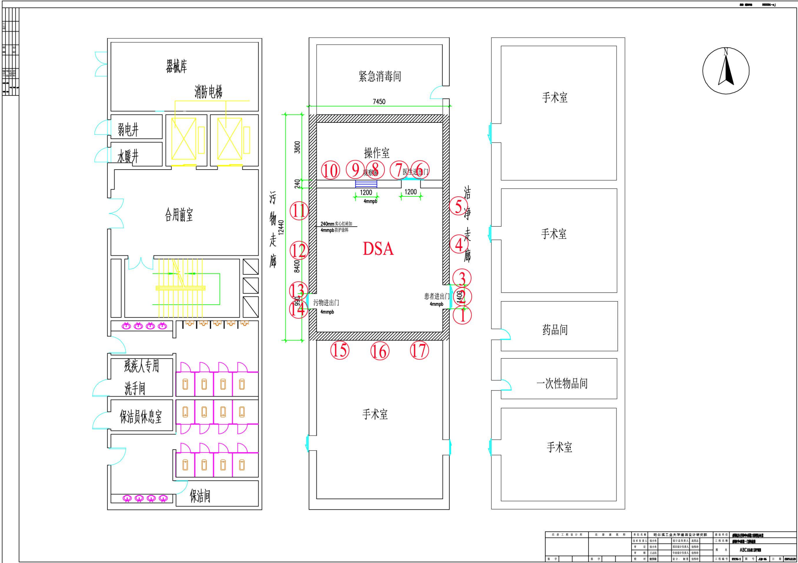
附图 4 DSA 手术室平面及采样点图
